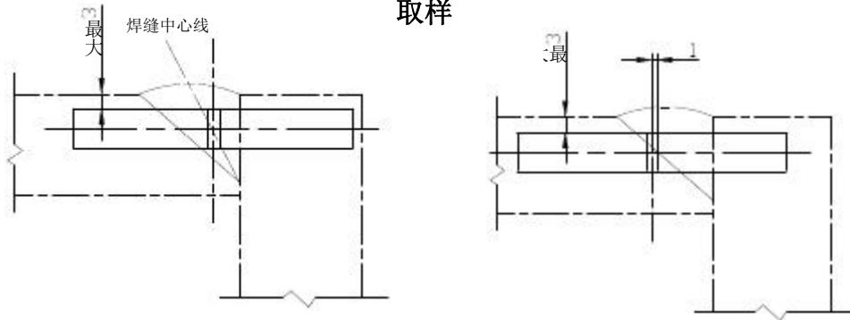
a) 焊缝金属冲击试样取样 b) 线外 1mm 冲击试样取样
