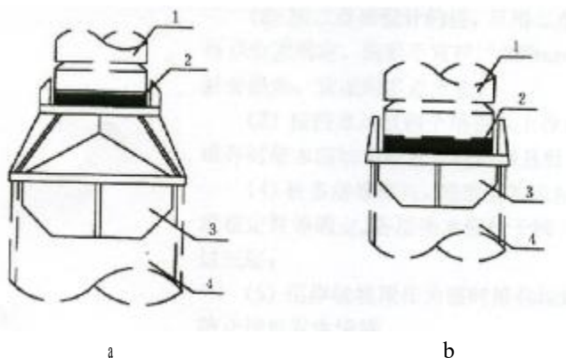
图 9.4.8 钢管桩锤击沉桩替打型示意图
