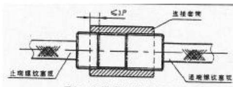
图 4.2.3 -15 套筒质量检验示意图
