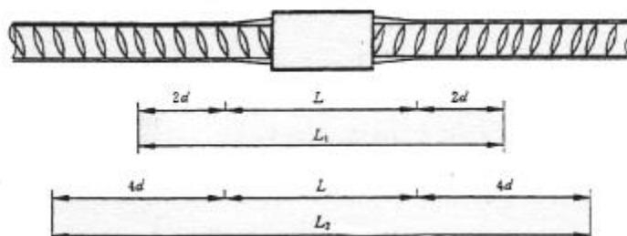
图 4.2.1 试件尺寸
