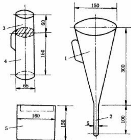
附图 C-2-1 粘度计(单位:mm) 1-漏斗;2-管子;3-量杯 200ml 部分;4-量杯 500ml 部分;5-筛网及杯
