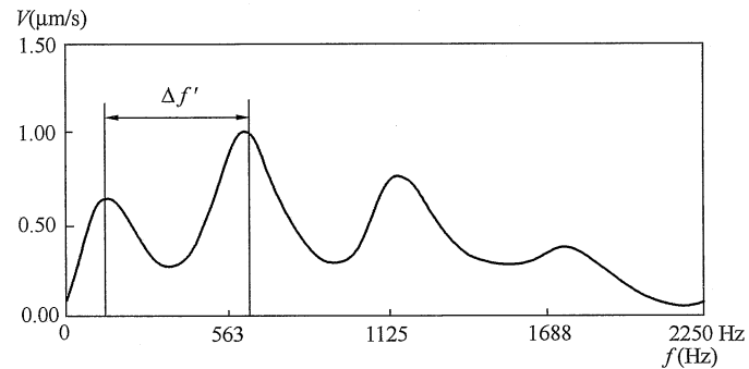
图 12.4.2-2 缺陷位置频域计算示意图
