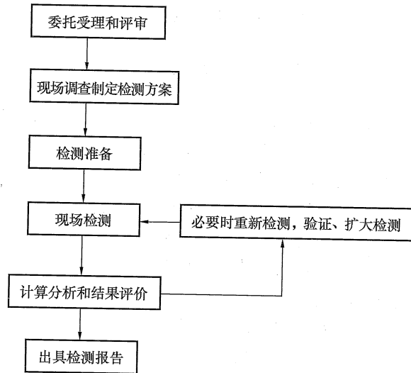
图 1 检测工作程序框图
