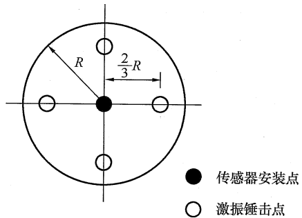
图 14 传感器安装点、锤击点布置示意图
